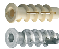
KBT, KBTM -kevytbetonitulpat
